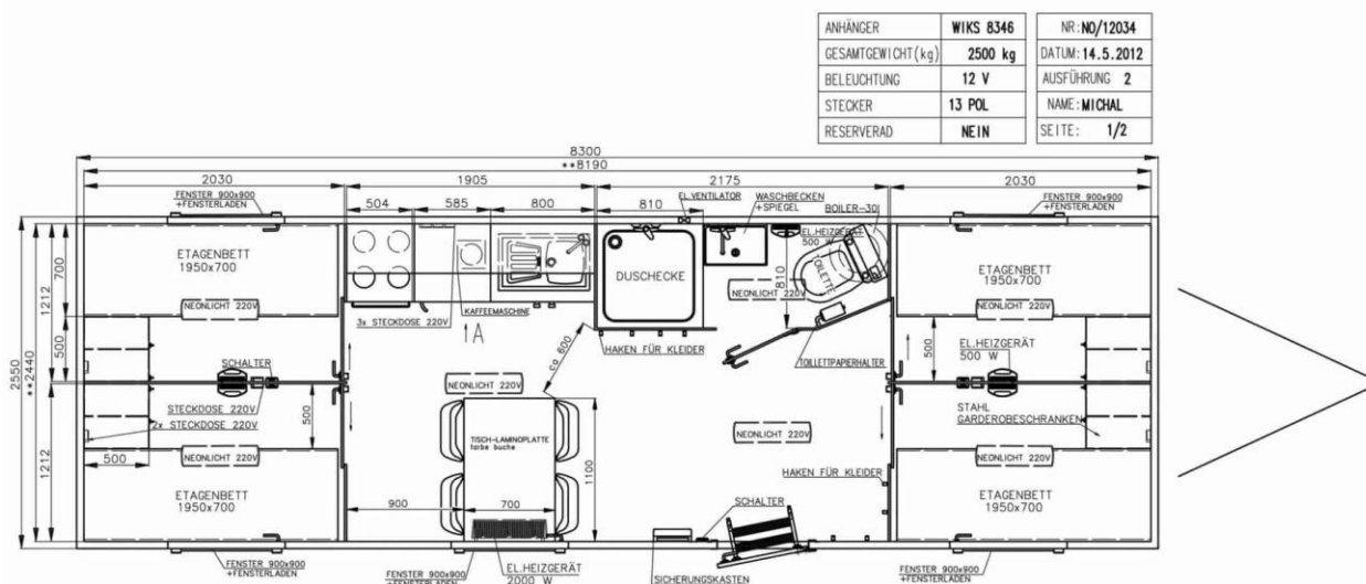
Teknisk tegning - Wiks Boligbrakke / Sovebrakke MOBI-8346
