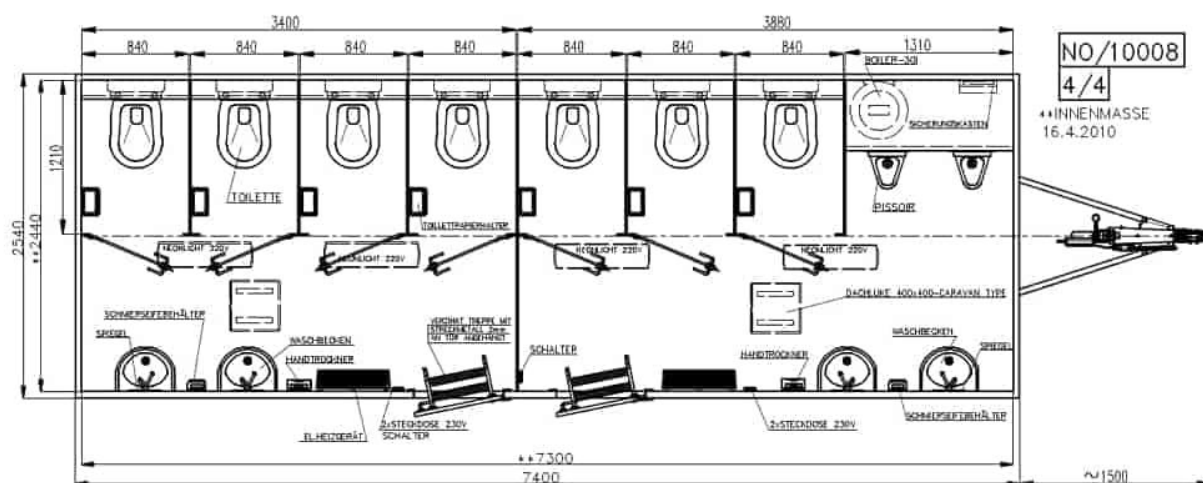
Teknisk tegning - Wiks Sanitærbrakke / Toalettbrakke MOBI-7374
