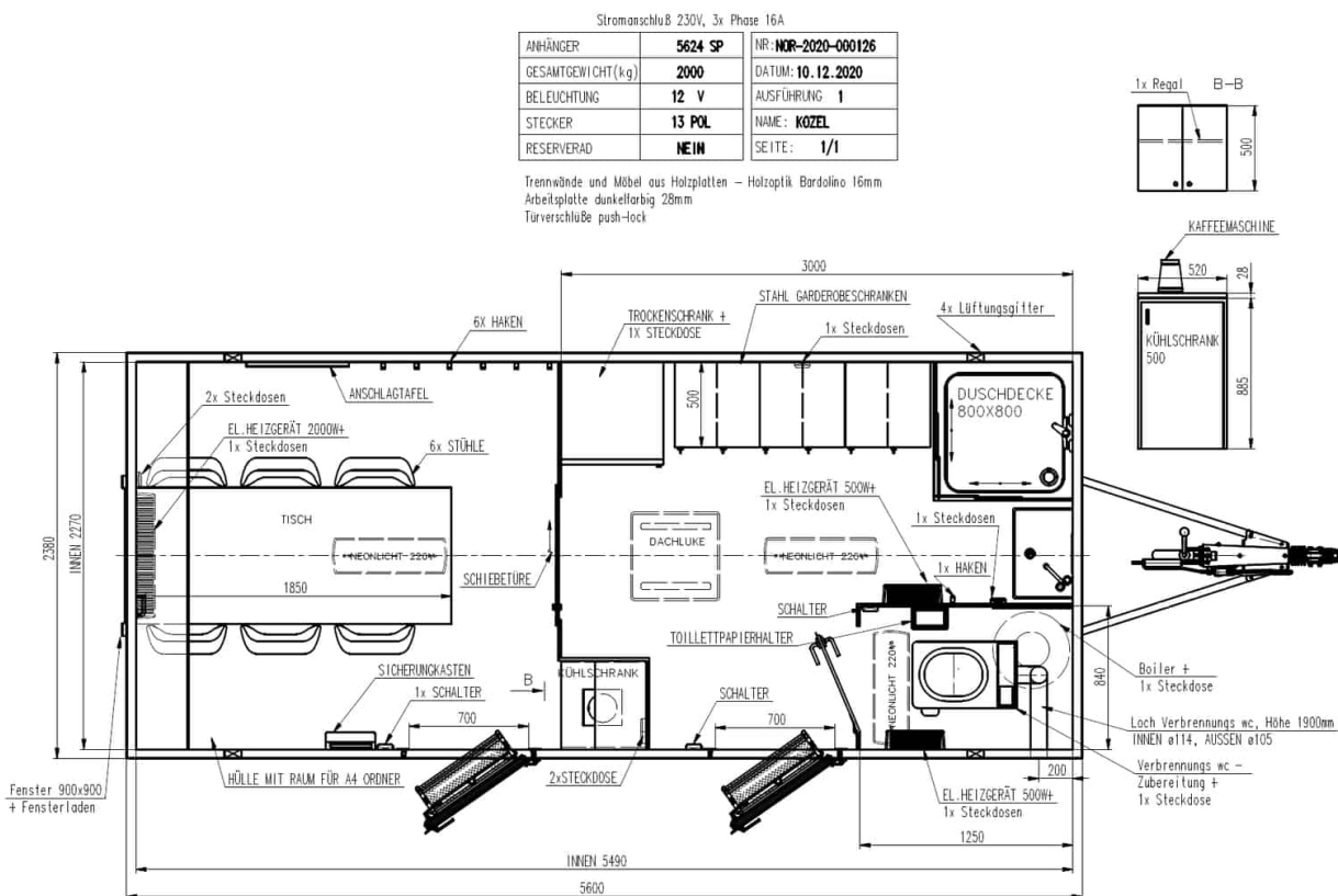
Teknisk tegning - Wiks Mannskapsbrakke MOBI-5624
