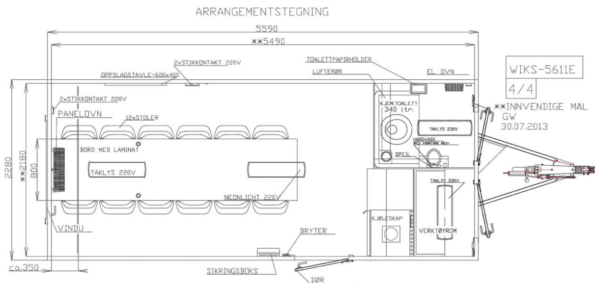
Teknisk tegning - Wiks Spisebrakke MOBI-5611E
