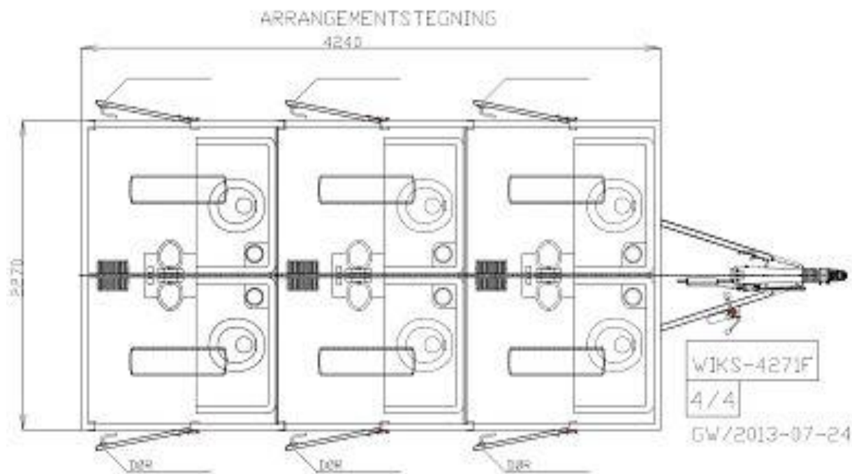
Teknisk tegning - Wiks Sanitærbrakke / Toalettbrakke 4271F
