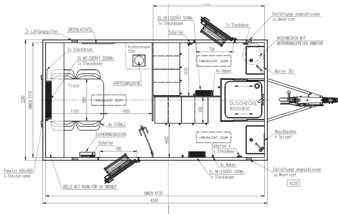
Teknisk tegning - Wiks Spezialvogn MOBI-4250
