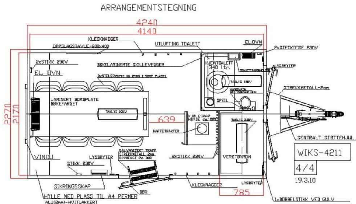
Teknisk tegning - Wiks Spisebrakke MOBI-4211E
