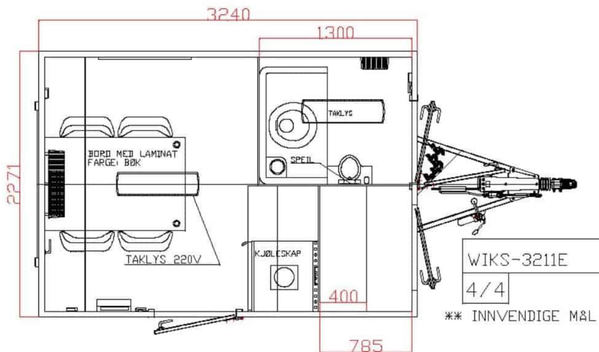
Teknisk tegning - Wiks Spisebrakke MOBI-3211E
