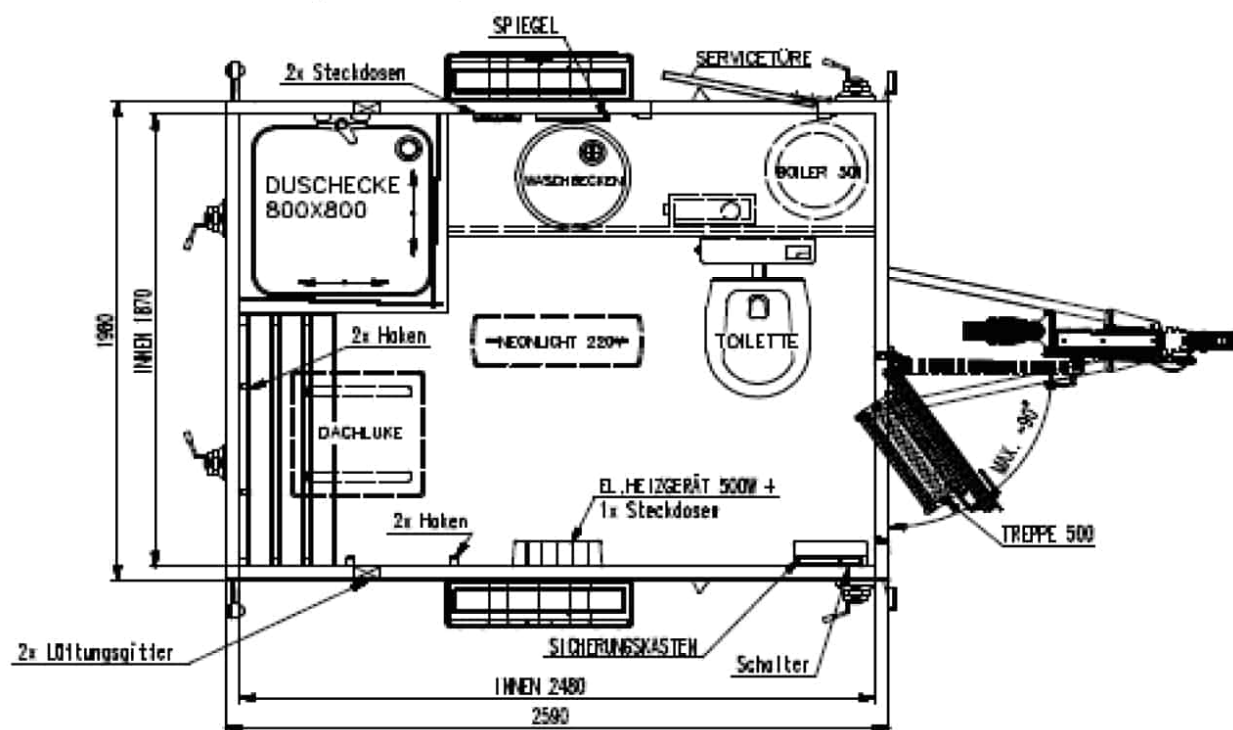
Teknisk tegning - Wiks Sanitærbrakke / Toalettbrakke MOBI-2482
