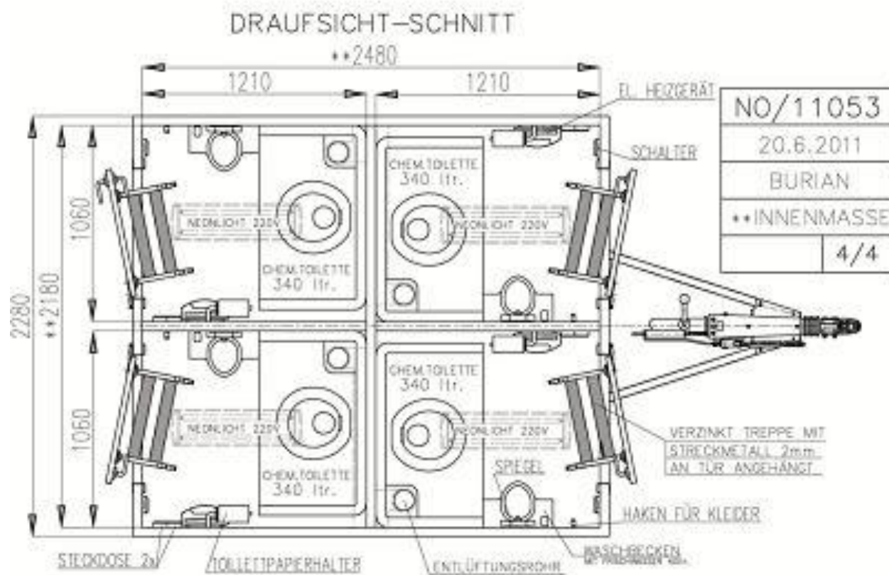
Teknisk tegning - Wiks Sanitærbrakke / Toalettbrakke 2473F
