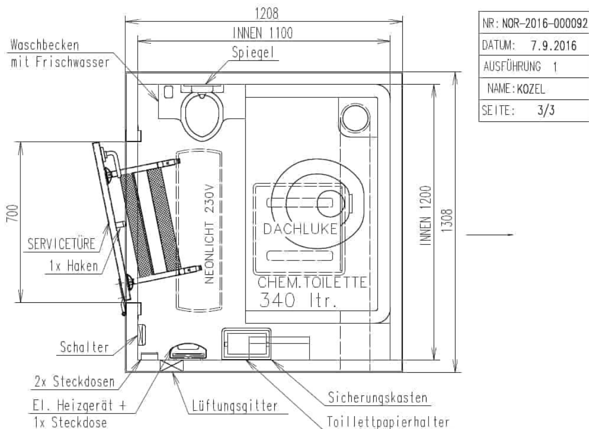
Teknisk tegning - Wiks Sanitærbrakke / Toalettbrakke MOBI-1073
